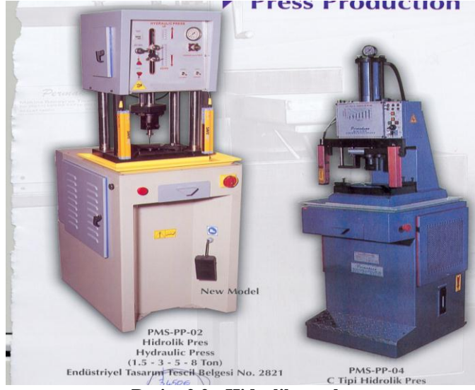
Resim 2.2: Hidrolik presler
