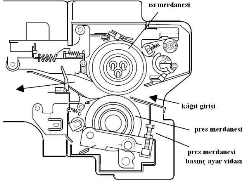
Şekil 1.9: Vida ayarlı pres merdanesi
