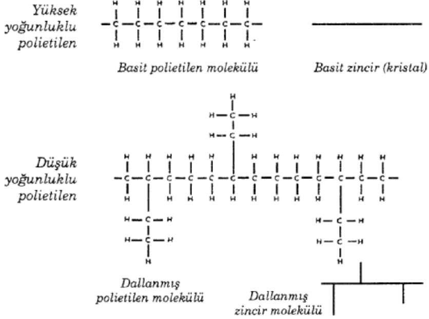
Şekil 2.4: Polietilen molekülleri
