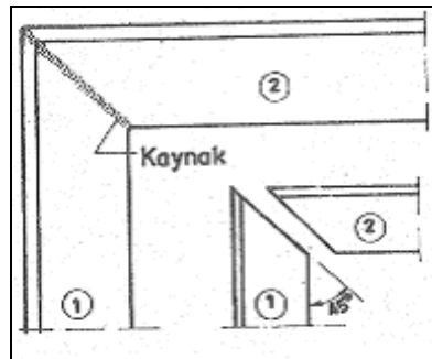
Şekil 1.6: 45° açılı keserek bükme
